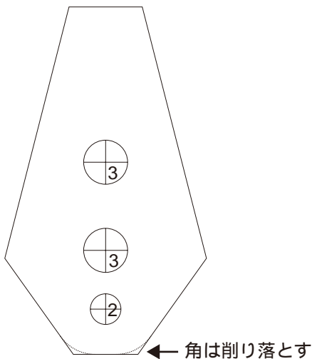
トゥイッチブレード (主にシュリンプ・ホッグ系)
